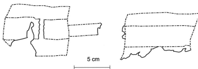
Abb. 168 Reste von zwei Besätzen aus Grab 39 (1966/27). Umrisszeichnung der erhaltenen Fragmente (Inv. HMB 1966.1721.13.a-b).
