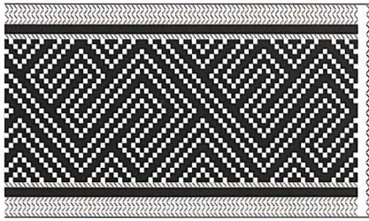
Abb. 238 Musterzeichnung des geometrischen Schlingmusters an der Brettchenborte der Pontifikalschuhe aus Grab 104 (1974/29).
