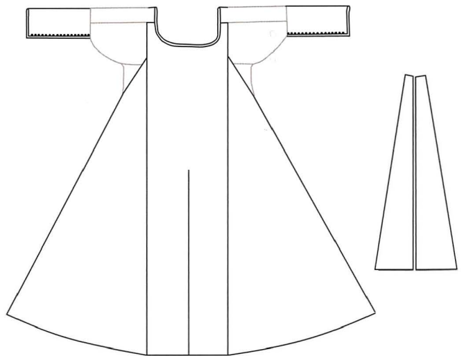
Abb. 246 Untergewand aus Grab 104 (1974/29). Rekonstruktionszeichnung.
