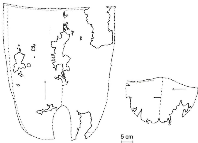
Abb. 132 Pontifikalstrümpfe aus Grab 6 (1907/04). Schnittrekonstruktion.
